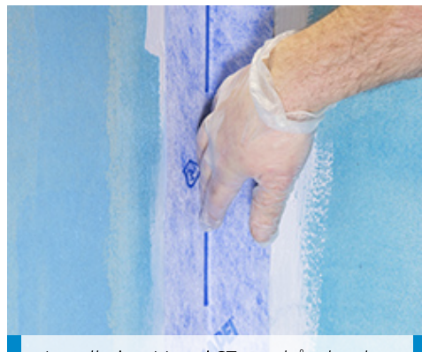
Installering Mapei ST tettebånd ved hjelp av Mapegum WPS, overgang vegg
